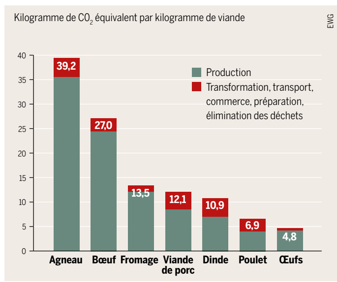
Émissions dues aux produits d'origine animale consommés aux USA
