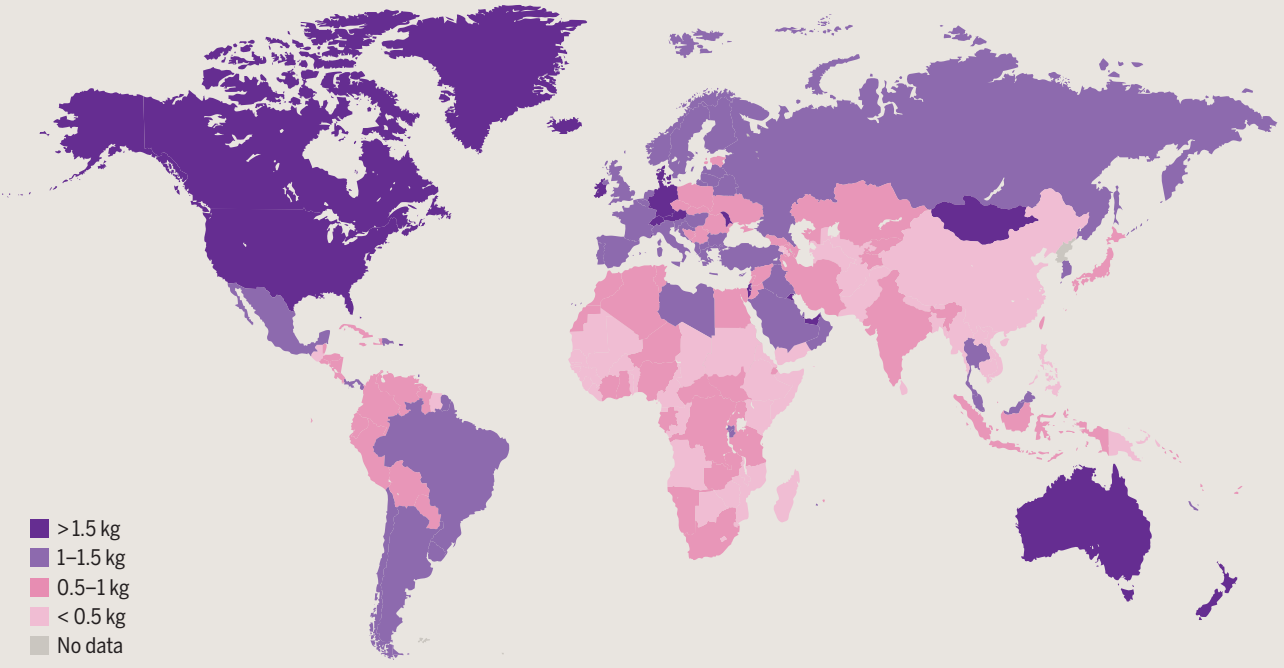
ABONDANCE ET EFFLUENCE Production de déchets par personne et par jour (2016)
