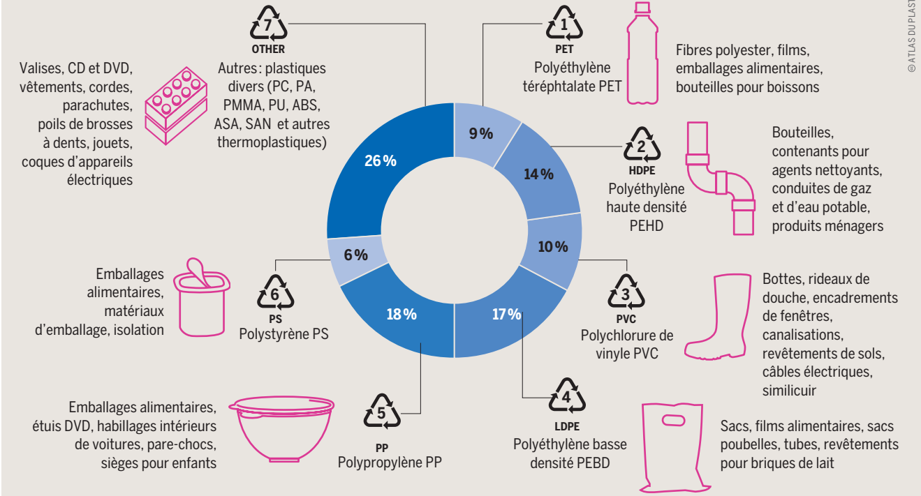
LE PLASTIQUE DANS TOUS SES ÉTATS Codes de recyclage définis par la Commission européenne et part de chaque type de plastique dans la production mondiale (2015)
